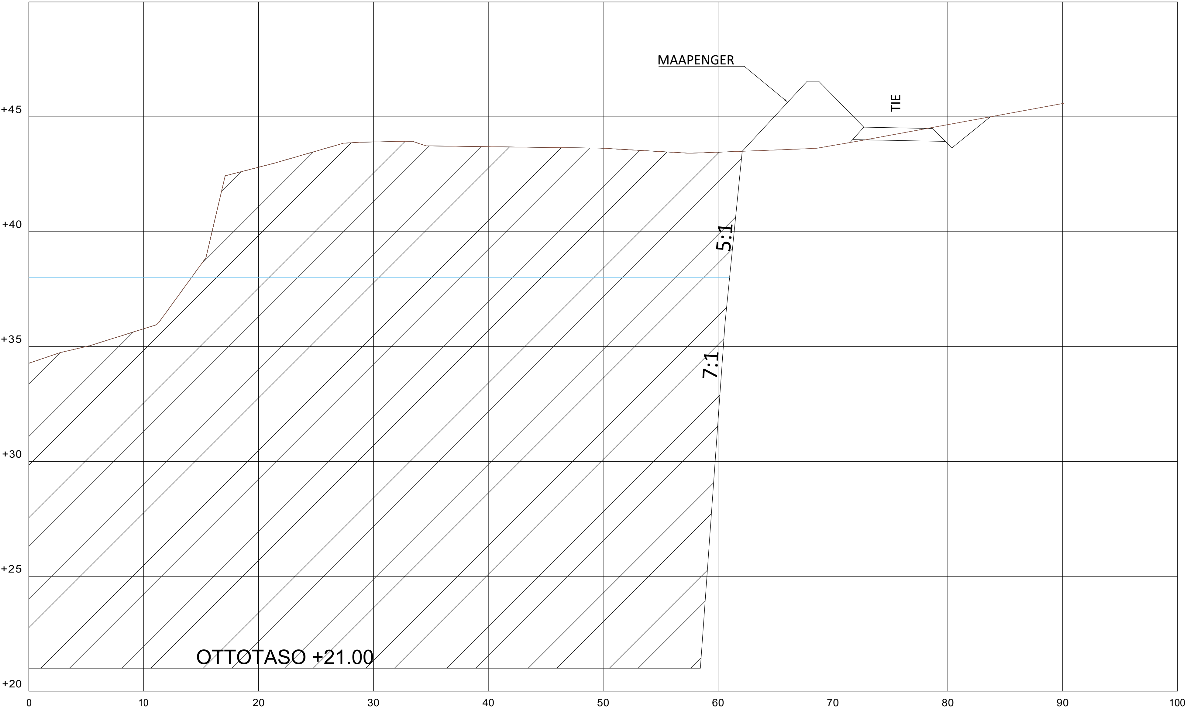
+50 LEIKKAUS B - B, 1:200/100
